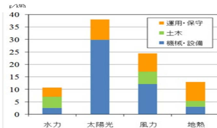
図2 再生可能エネルギーの CO 2 排出量原単位
